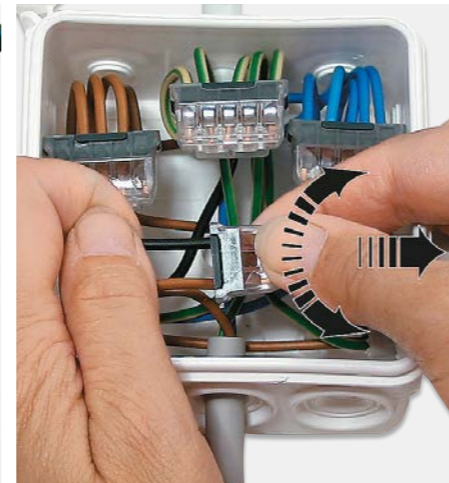
Lösen des Leiters durch Drehen und Ziehen Release the wire by twisting and pulling
